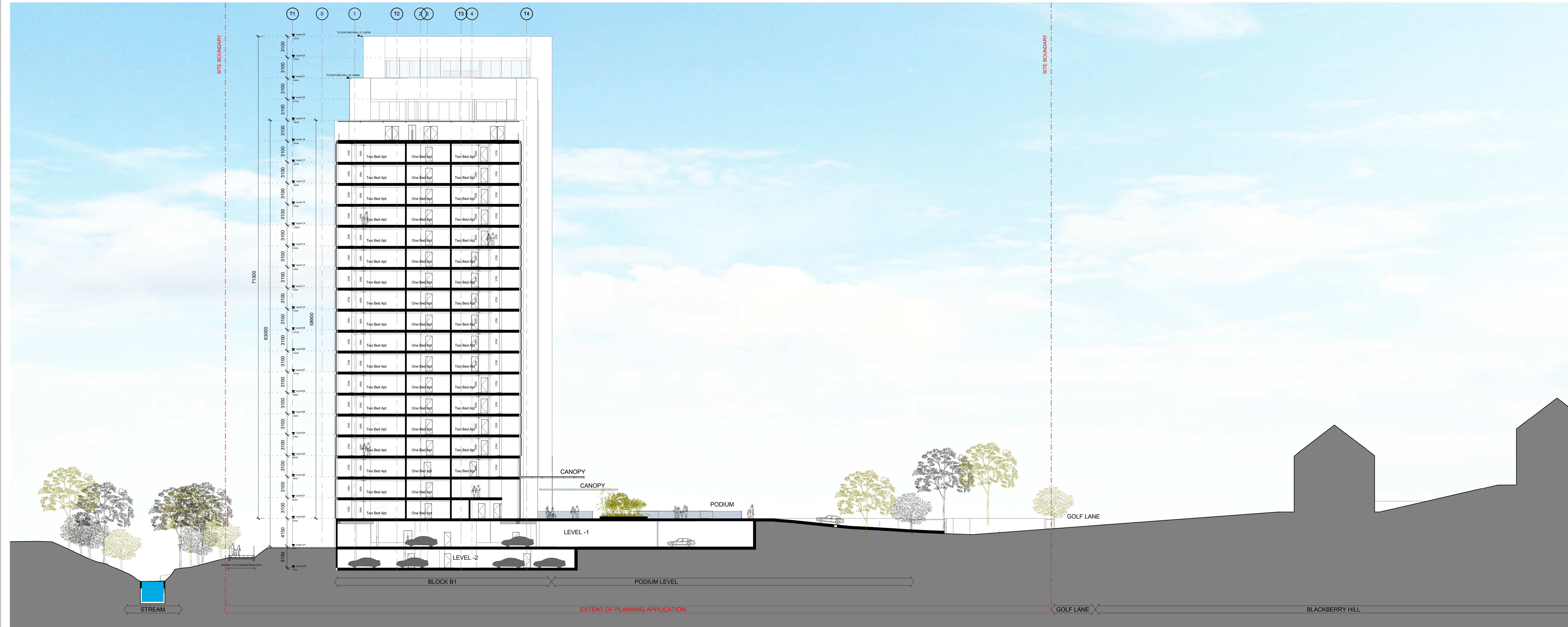
2 Site Section 02 1 : 250
