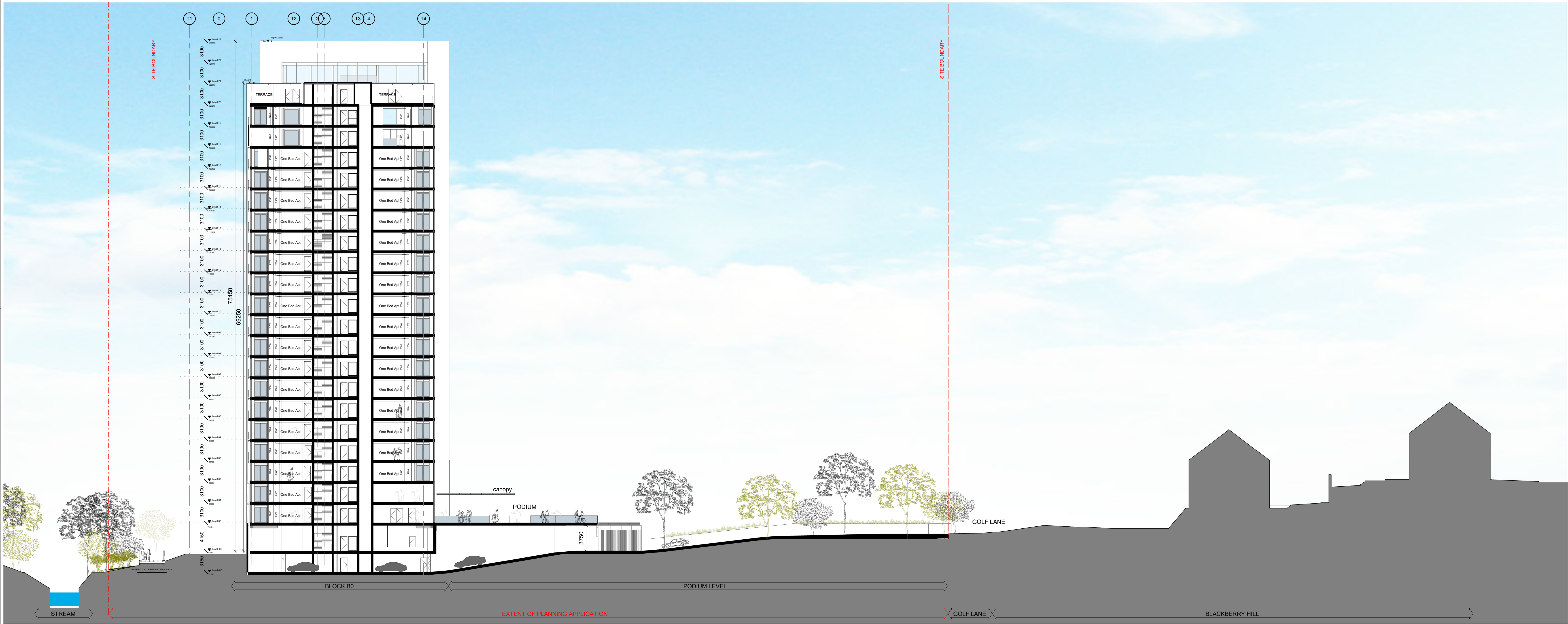
1 Site Section 01 1 : 250
